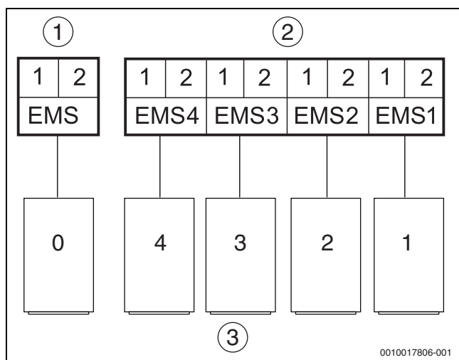
Мал. 4 Клеми EMS
