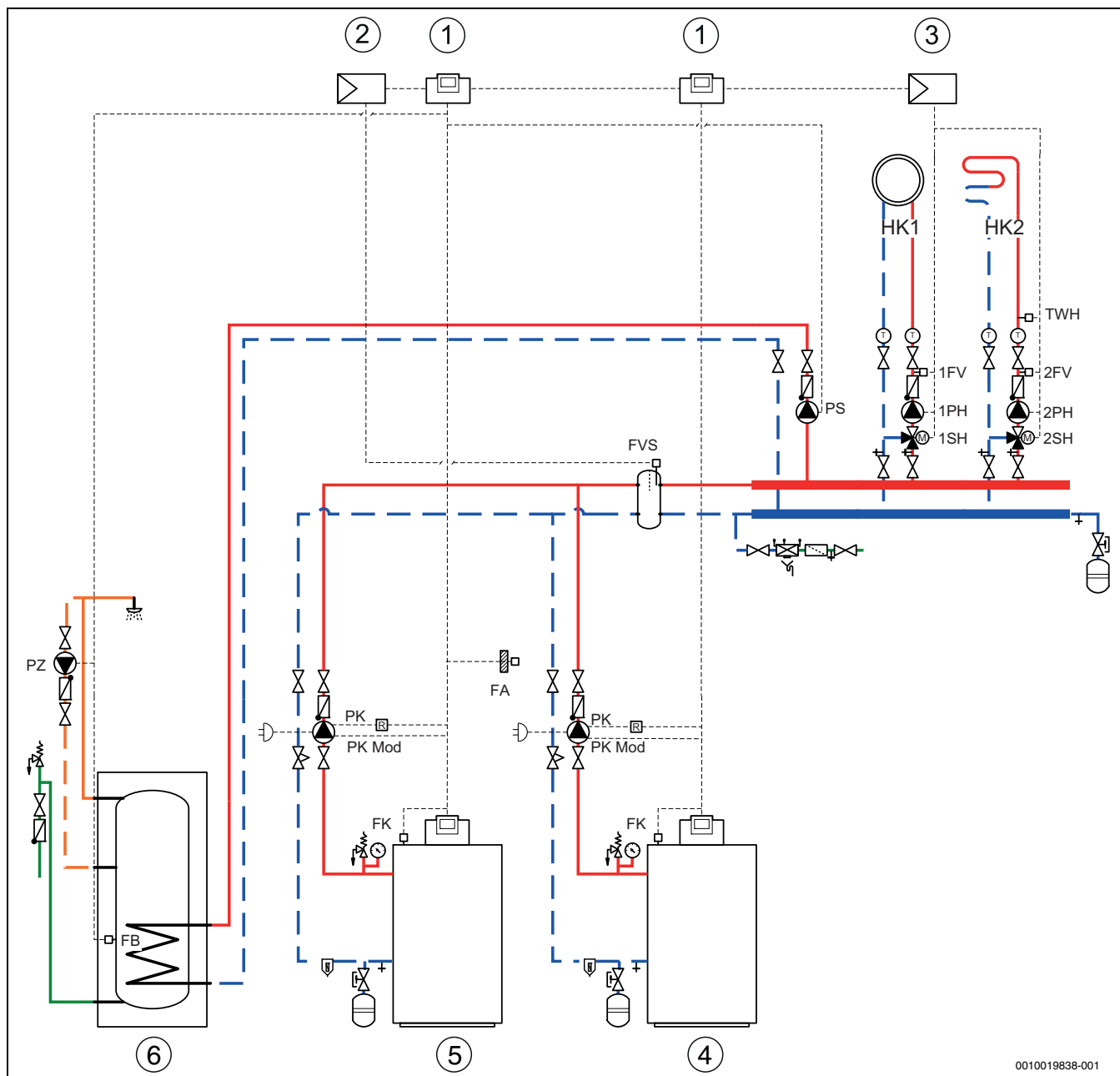
Мал. 26 Теплогенератор зі штекером
