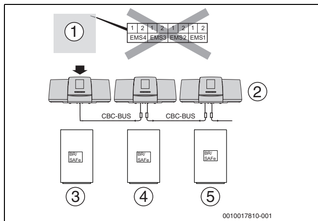
Мал. 5 Багатокотлова установка з Logamatic 5000/Control 8000
