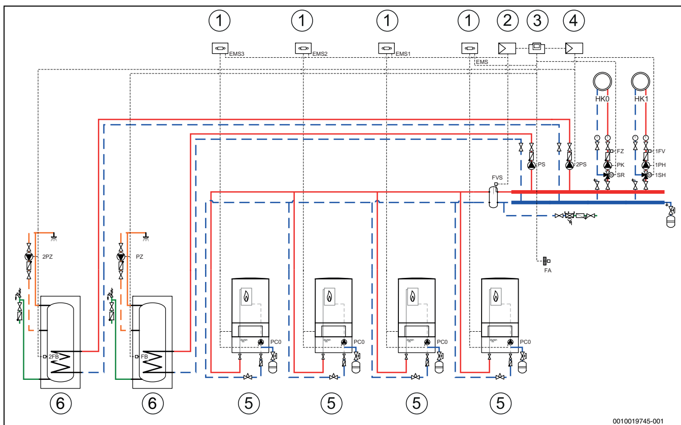
Мал. 20 Гідравлічна схема 4: паралельне підключення настінних конденсаційних котлів EMS з гідравлічною стрілкою
