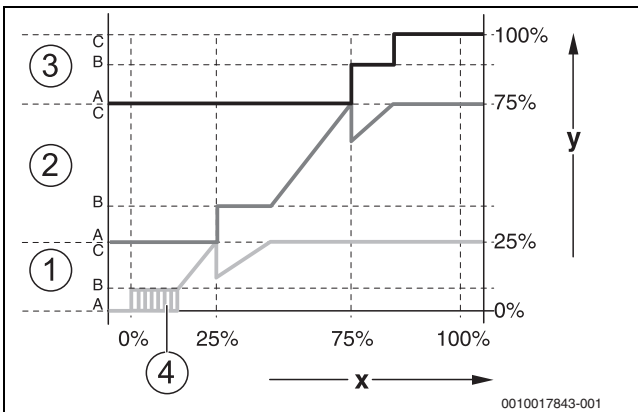
Мал. 14 Діаграма послідовного режиму експлуатації
