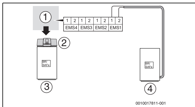
Мал. 6 Багатокотлова установка із системою керування EMS
