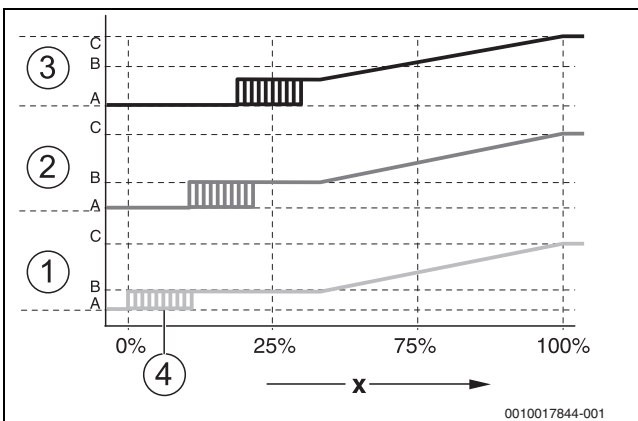
Мал. 15 Діаграма паралельного режиму експлуатації
