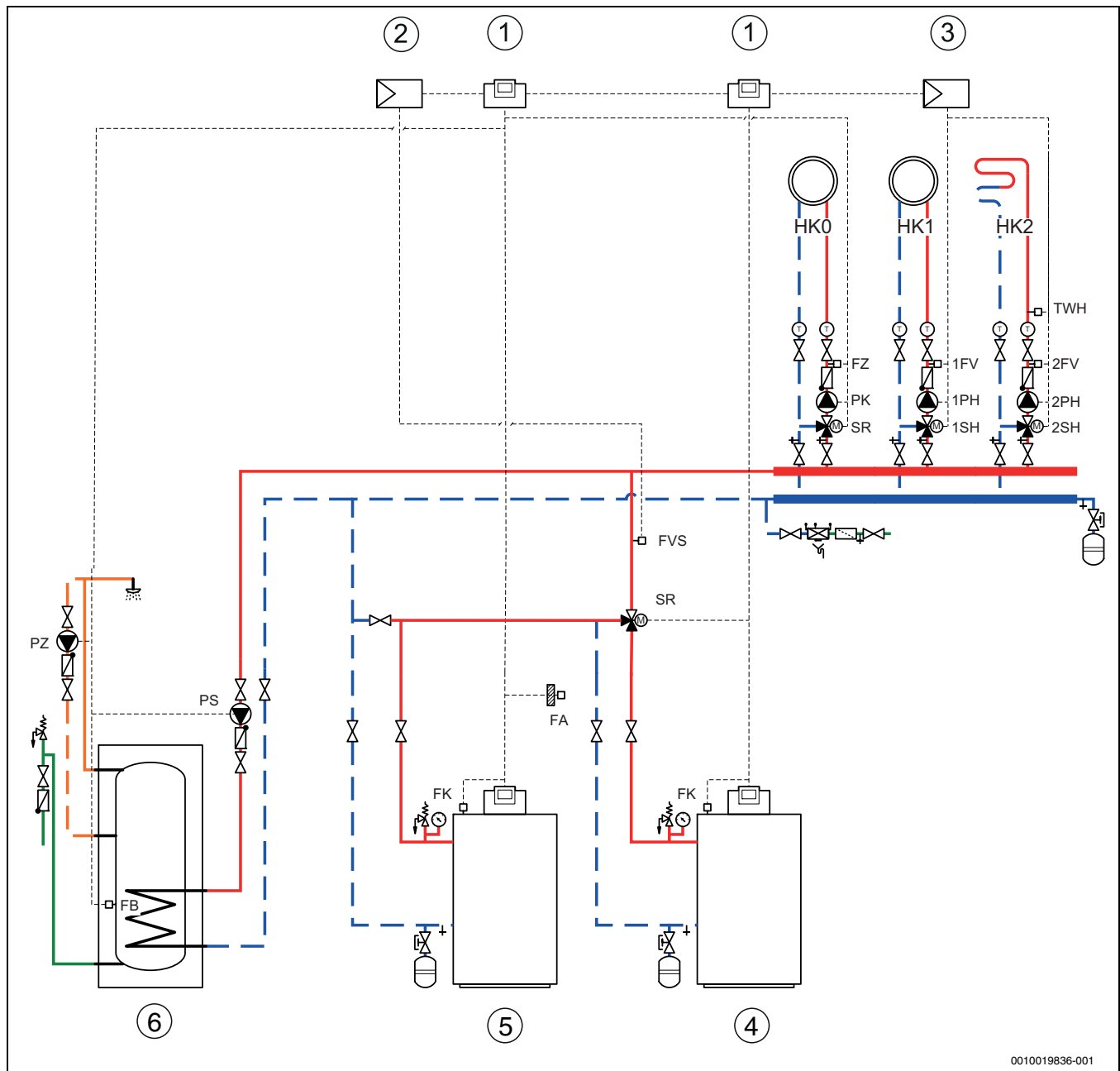
Мал. 25 Гідравлічна схема 8: змішаний каскад із теплогенератором зі штекером
