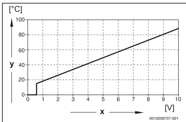
Мал. 9 Вихід 0–10 В Температура
