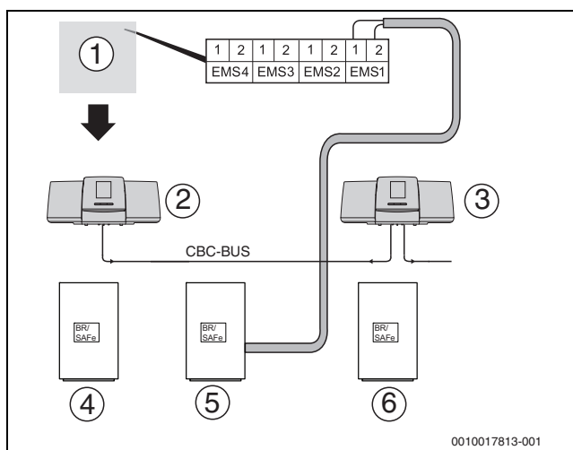
Мал. 7 Багатокотлова установка з Logamatic 5000/Control 8000 і системою керування EMS
