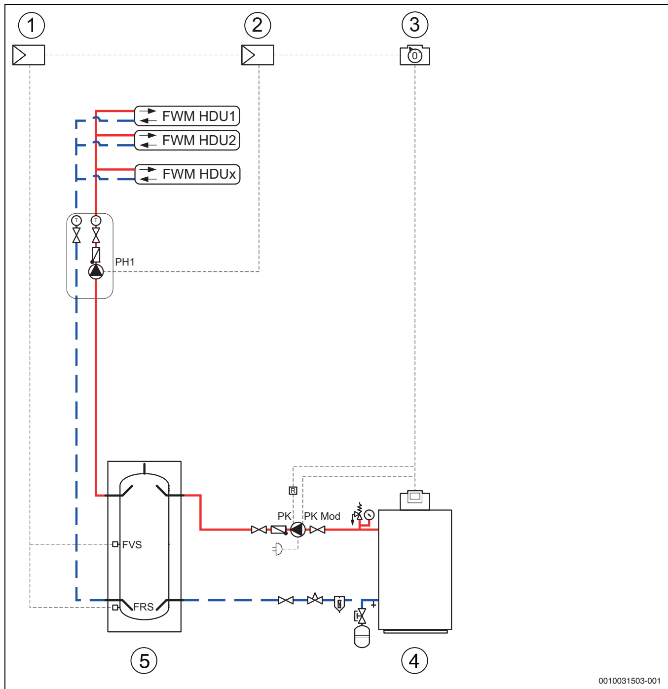
Мал. 27 Теплогенератор із блоком керування пальником SAFe
