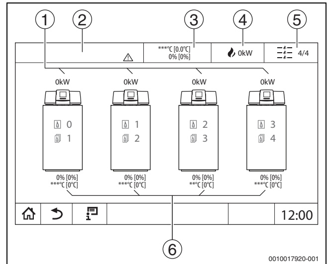
Мал. 1 Каскад теплогенераторів
