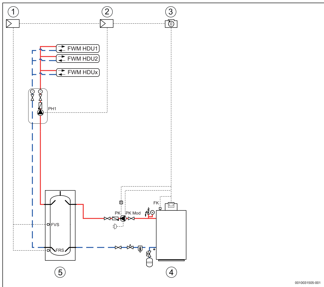
Мал. 28 Теплогенератор з окремим пальником, попередньо налаштованим на заводі
