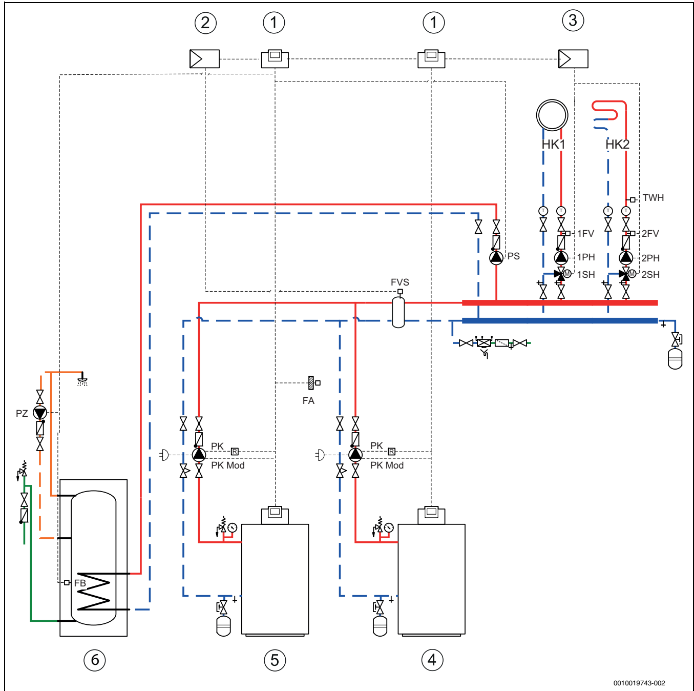
Мал. 19 Гідравлічна схема 2: теплогенератор із блоком керування пальником SAFe та гідравлічною стрілкою/теплообмінником: паралельне підключення
