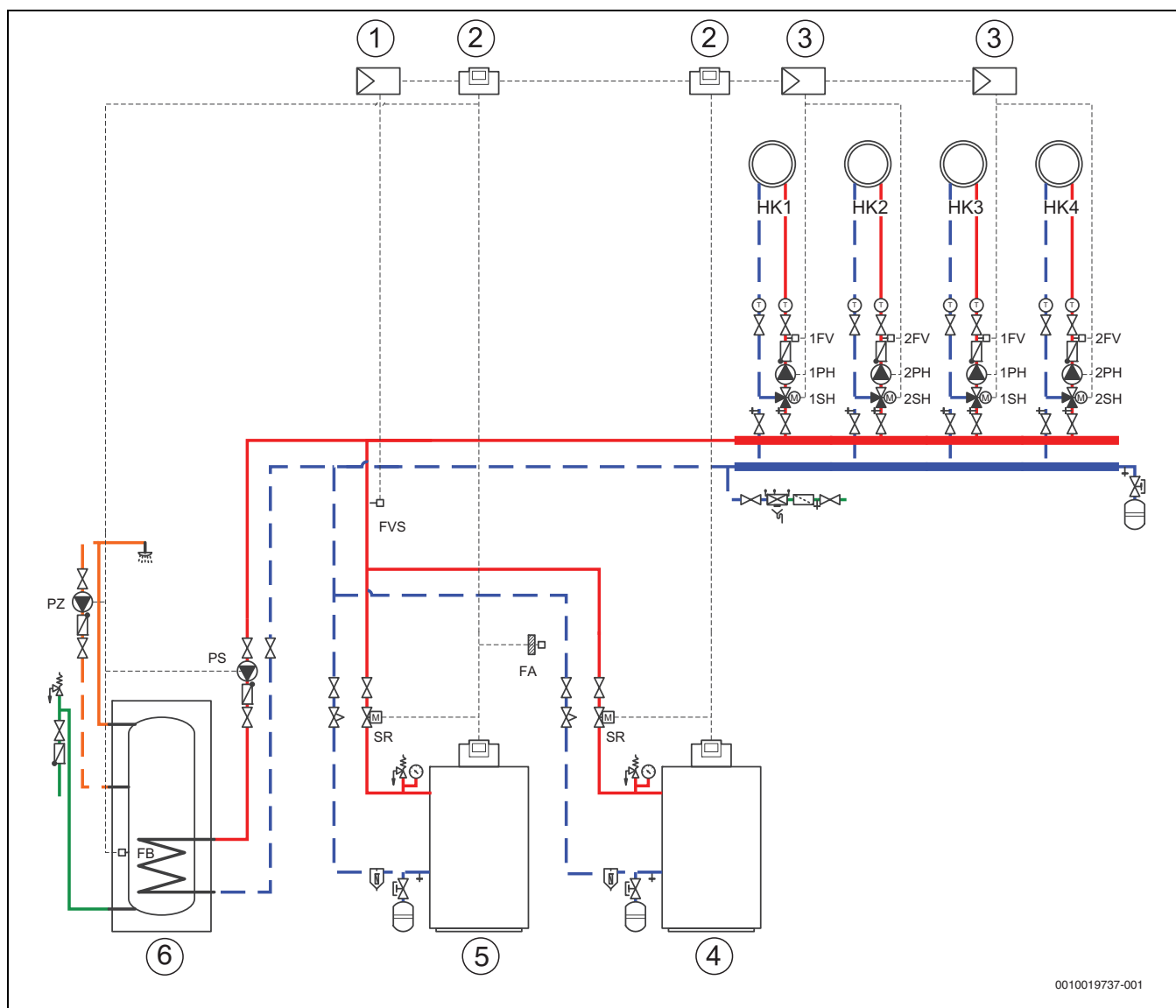
Мал. 18 Гідравлічна схема 1: теплогенератор із блоком керування паливом SAFe – паралельне підключення
