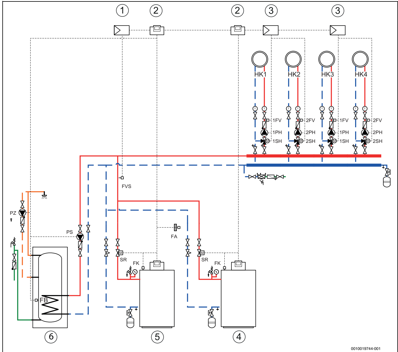
Мал. 21 Гідравлічна схема 3: теплогенератор зі штекером
